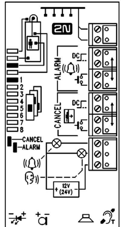
Obrázek 2.7 Nastavení adresy pro Hlásku – kabinu univerzál
