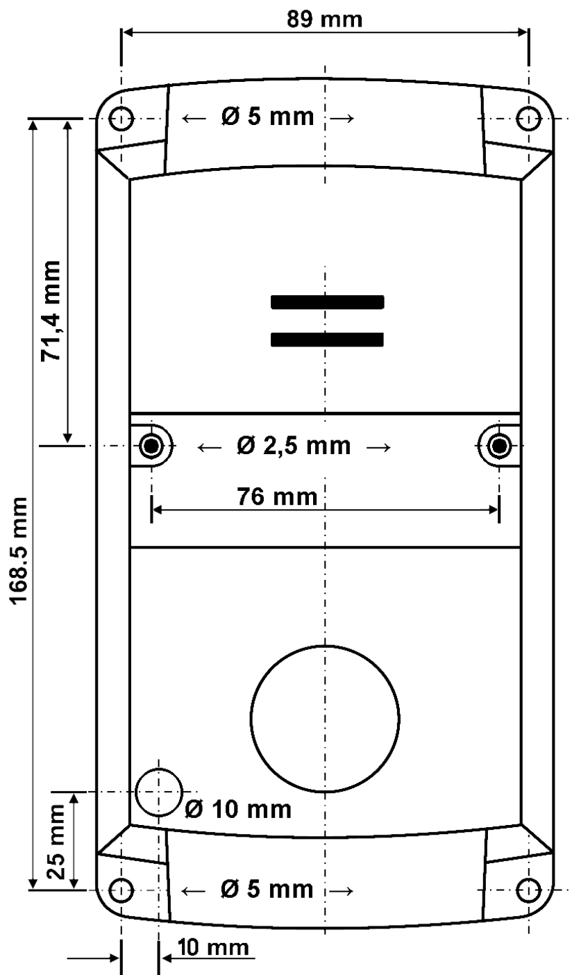
Obrázek 2.12 Rozměry montážních otvorů pro hlášku – kabinu kompakt
