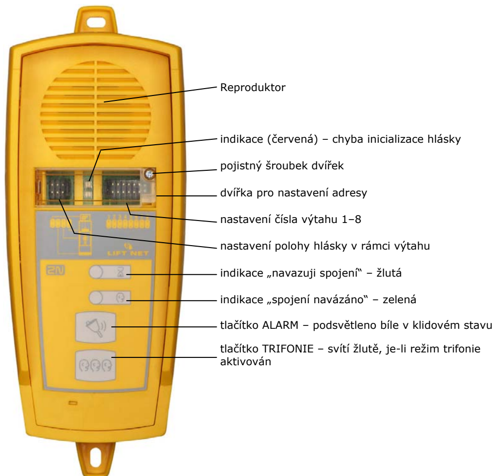
Obrázek 2.17 Vyobrazení hlášky v šachtě s popisem indikačních prvků
