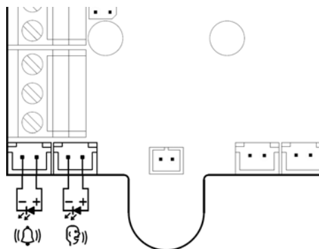
Obrázek 2.9 Alternativní zapojení indikačních prvků pro Hlásku – kabinu univerzál
