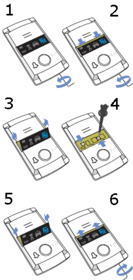
Obrázek 2.11 Nastavení adresy pro Hlášku – kabina kompak
