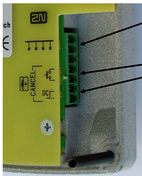
Obrázek 2.13 Konektory na Hlásce – kabině kompakt
