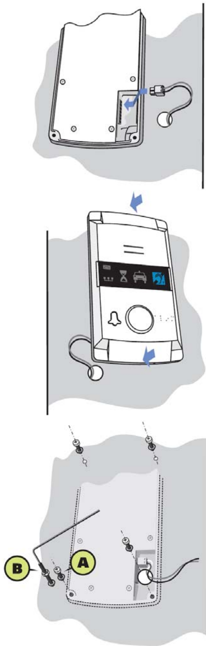
Obrázek 2.14 Montáž hlásky – kabiny kompakt
