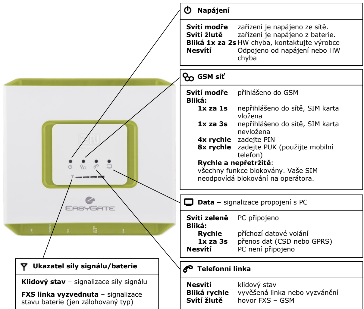
Obrázek 2.1 Indikační prvky EasyGate
