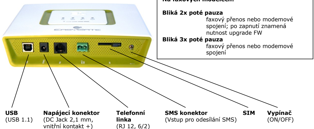
Obrázek 2.2 Konektory EasyGate
