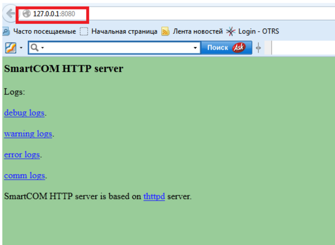
Obrázek 5. Logy serveru
